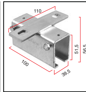
Soffit bracket KKKL-102
