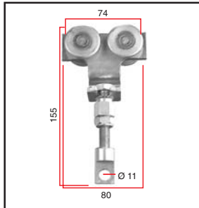
Letkunripustin pyörästä LP/4-102
