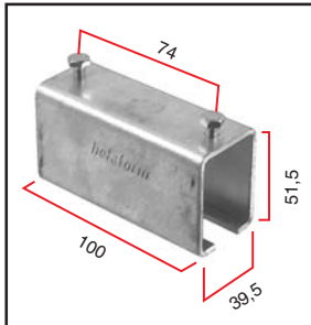
Liitoskotelo LK-102 pituus 100 mm
