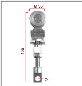
Letkunripustin pyörästä LP/2-102
