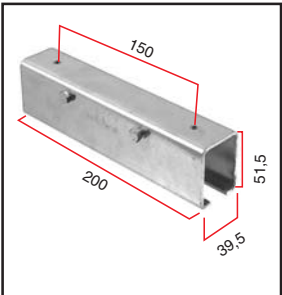
Liitoskotelo LK-102 pituus 200 mm
