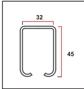
Kisko K-102, profiilikuva
