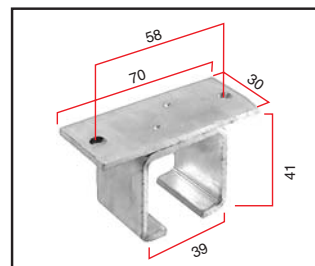
Потолочный кронштейн ККК-100 литой
