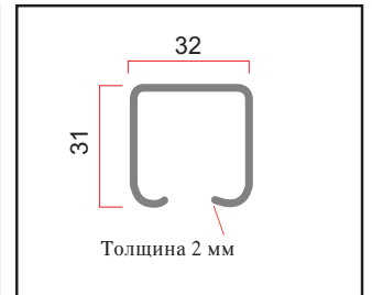
Профиль К-100 Грузоподъемность 100 кг, стандартная длина 6 м
