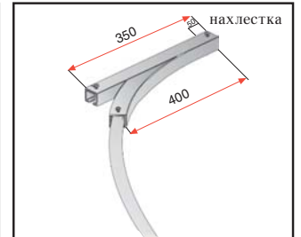
Рельсовый переход (стрелка)
