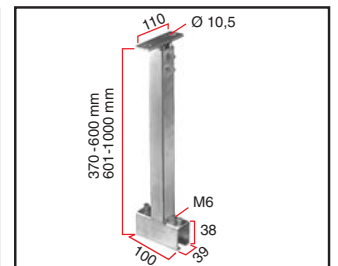
Потолочный кронштейн KKS-100, 370-600мм/601-1000 мм, регулируемый
