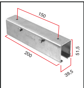
Соединительная деталь LK-102, длина 200 мм
