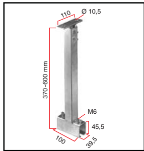
Потолочный кронштейн ККС-102
