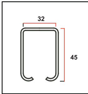
Профиль К-102
