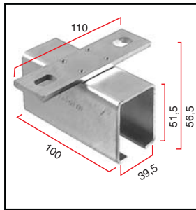
Потолочный кронштейн ККК-102
