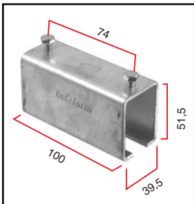
Соединительная деталь LK-102, длина 100 мм
