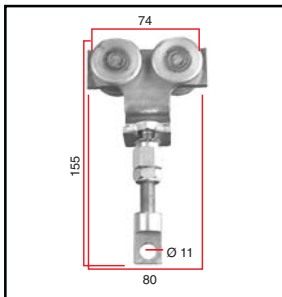
Ролик для шлангового хомутка LP/4-102
